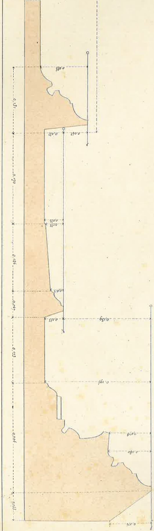
COUPE
