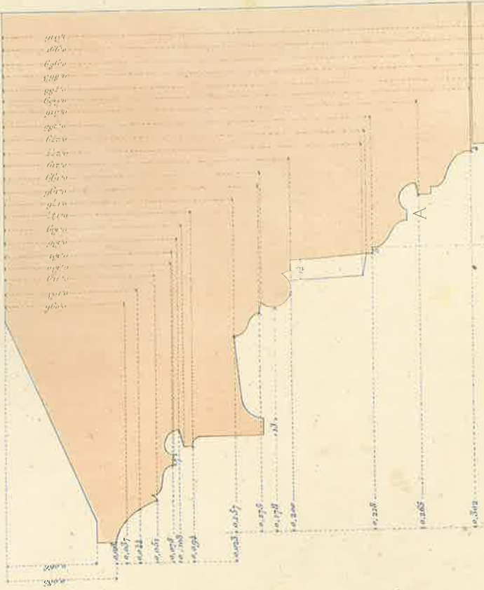
DETAIL A. \frac{1}{2} Grand f. d'Exécution.
