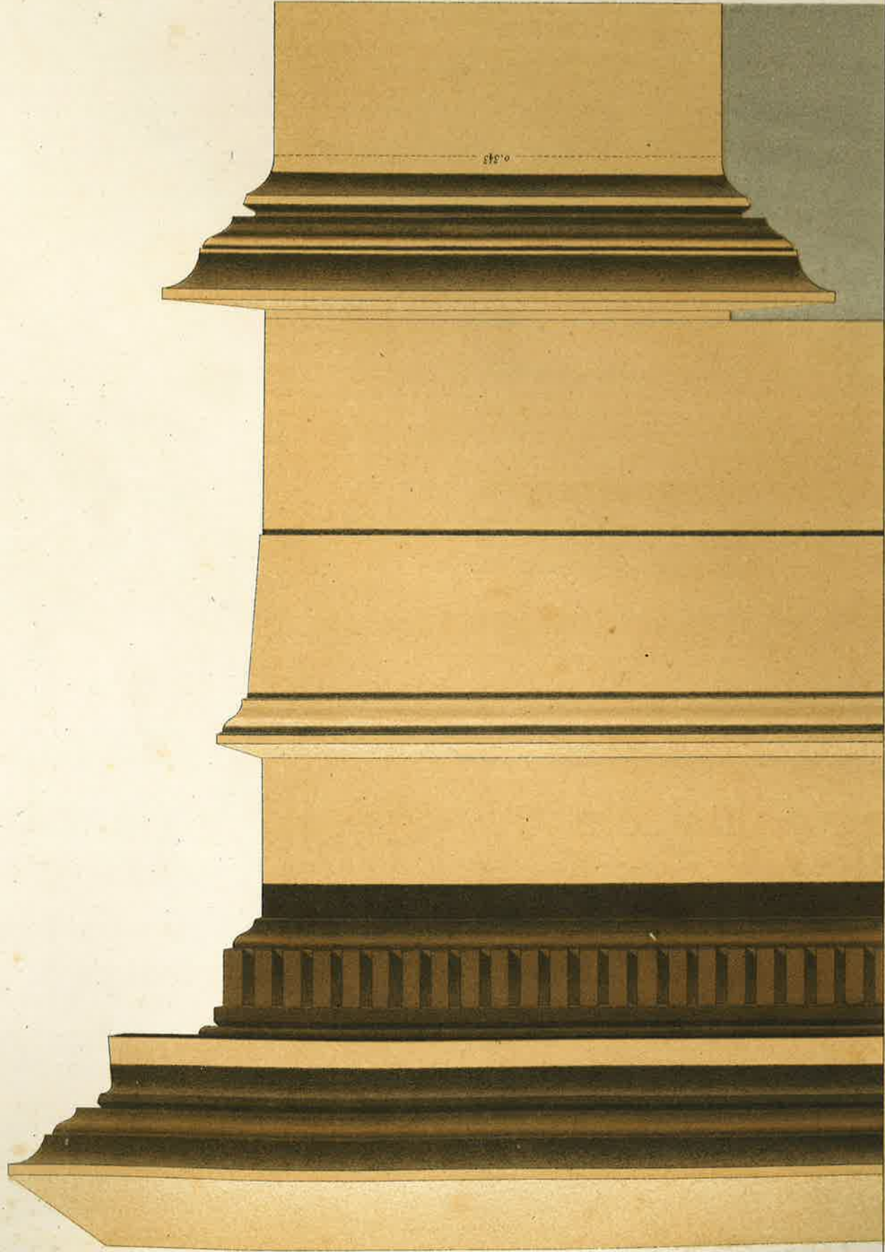
ENTABLEMENT Echelle de 0.25 e p.m.
