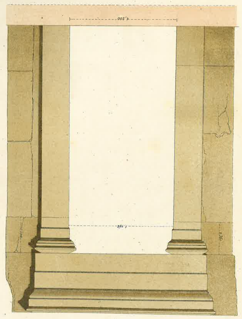
ELEVATION DE LA PORTE A DU PLAN Echelle de 0 m 04 e p r mètre
